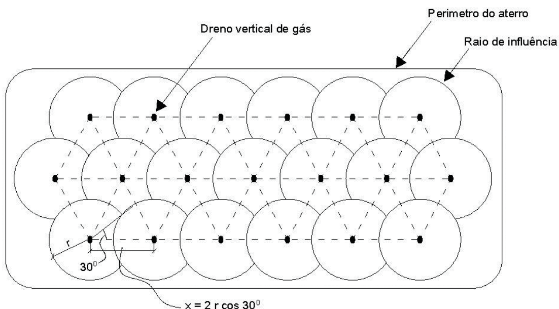
Figura 7 – Detalhe de sistema de drenagem (exemplo)
