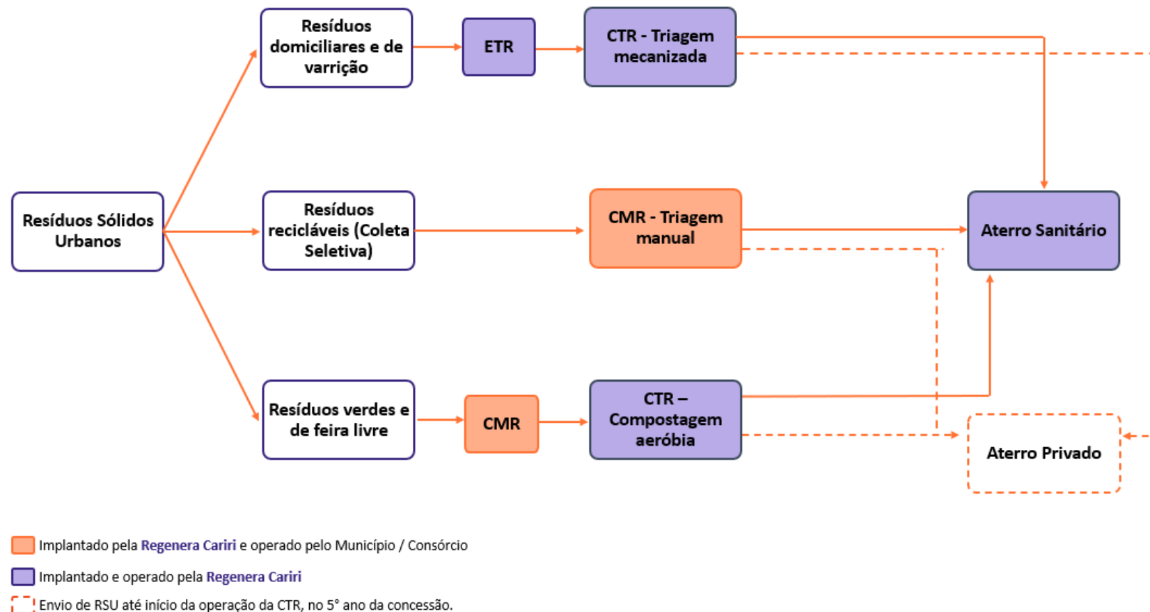
Figura 4 – Fluxograma das tecnologias que serão implantadas na CTR.
