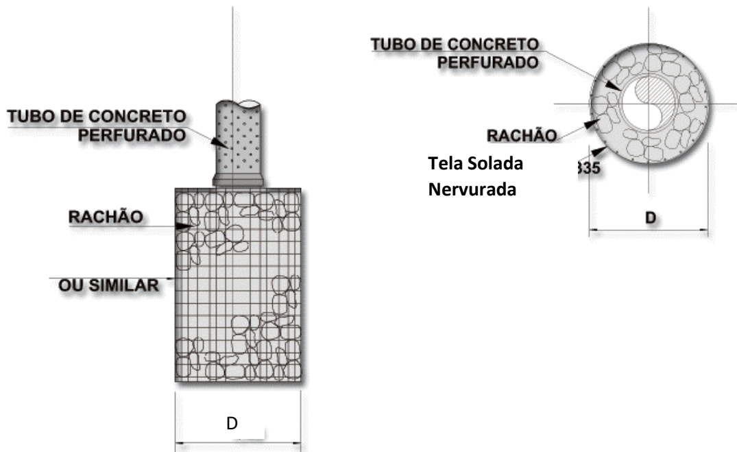
Figura 8 – Detalhe dreno de gás.
